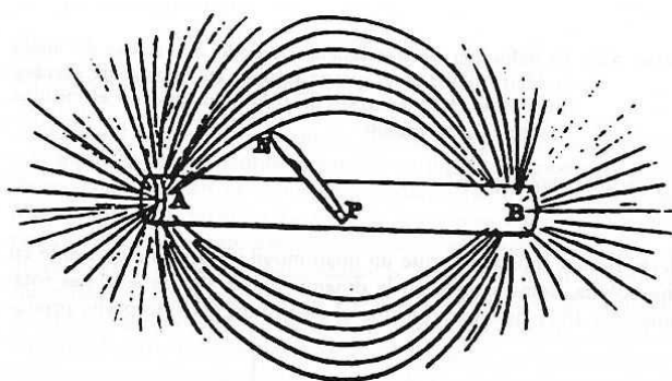
Figura 1.- Primer dibujo publicado por Faraday, en 1831, de las curvas magnéticas que rodean a un imán de barra.
