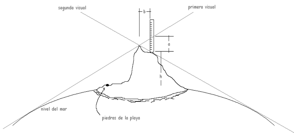
Figura1.- Cálculo del radio terrestre según la descripción del Método de Gerwer.
