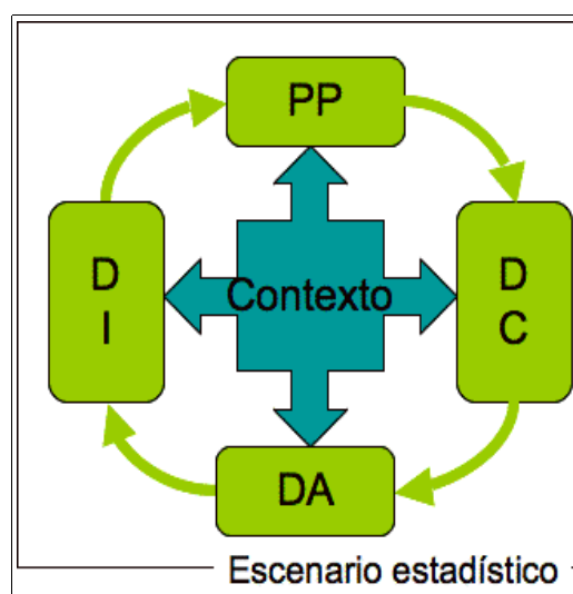
Figura 2.- Escenario estadístico, contexto y procesos.
